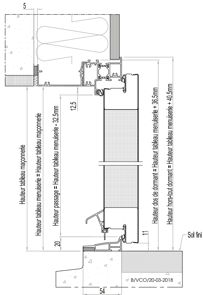
Coupe verticale
