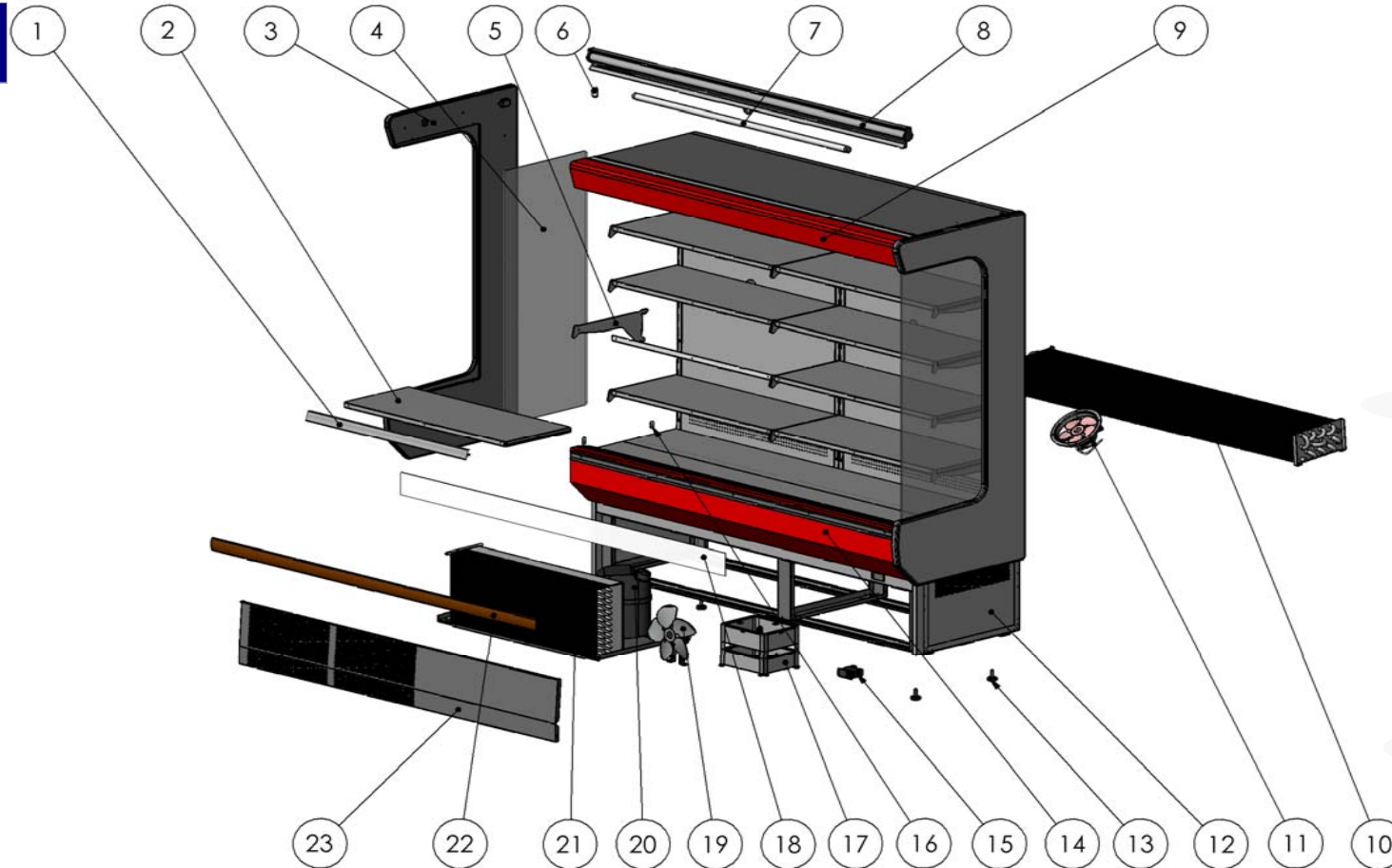
CM6- VITRINA ALTA. TALL DISPLAY UNIT
