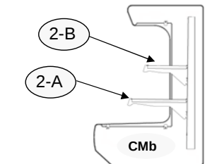
CMb6- VITRINA BAJA. LOW DISPLAY UNIT
